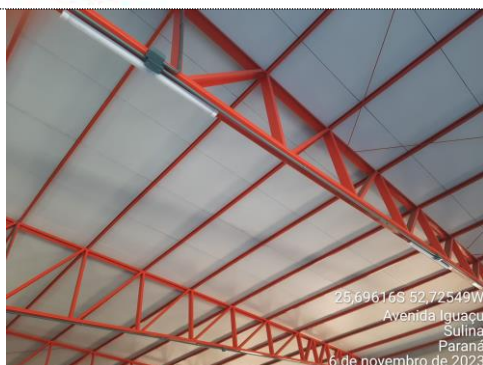
FOTO 23 ITEM 8.7: ELETRODUTO RÍGIDO ROSCÁVEL, PVC, DN 25 MM (3/4"), PARA CIRCUITOS TERMINAIS, INSTALADO EM FORRO - FORNECIMENTO E INSTALAÇÃO. AF_12/2015 MEDIDO: 73,50%
