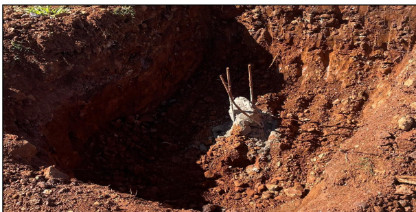
5 | ESCAVAÇÃO DOS BLOCOS APOS A CONCRETAGEM DAS ESTACAS
